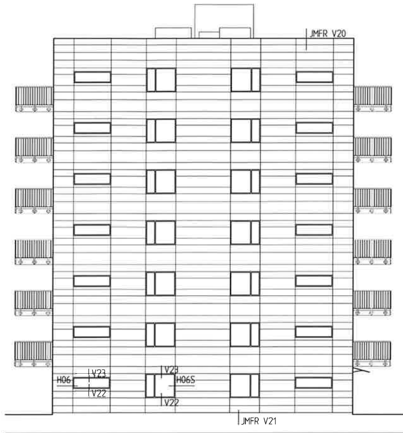
HUS 7 FASAD MOT NORR
