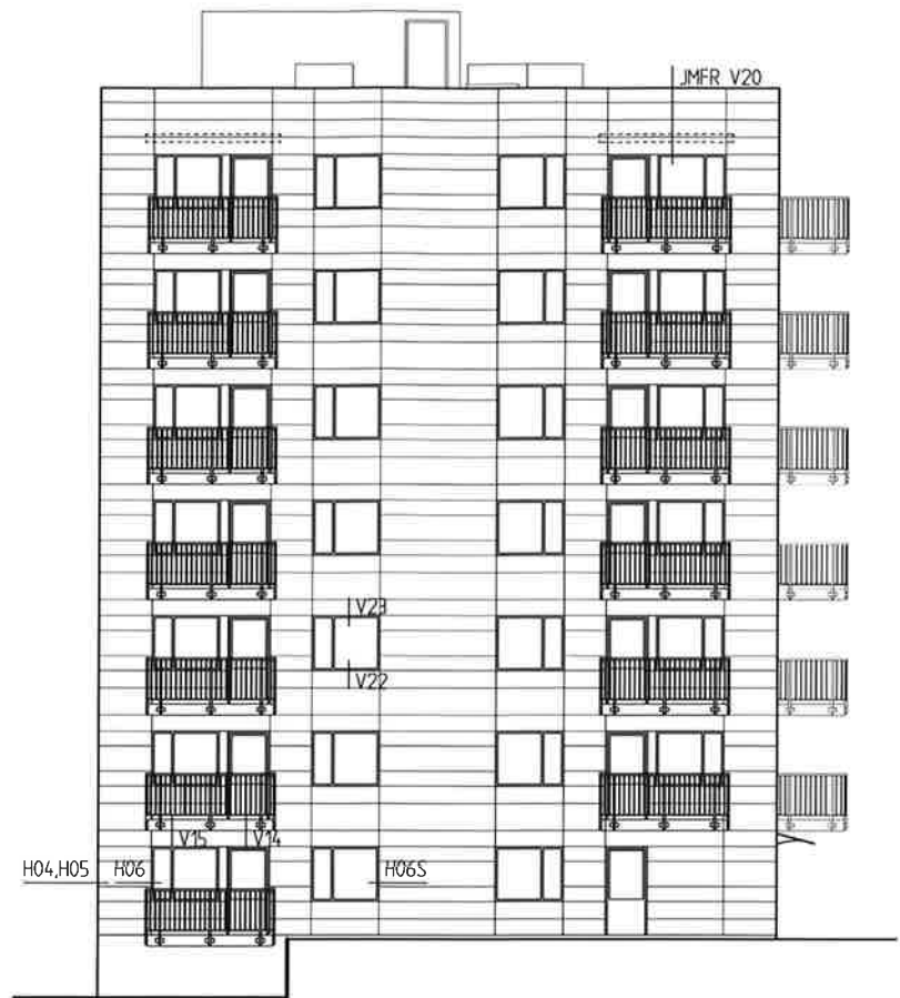
HUS 5 FASAD MOT NORDVÄST
