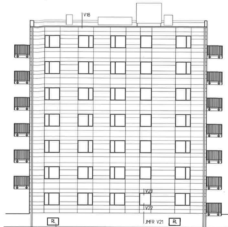
HUS 5 FASAD MOT NORDÖST
